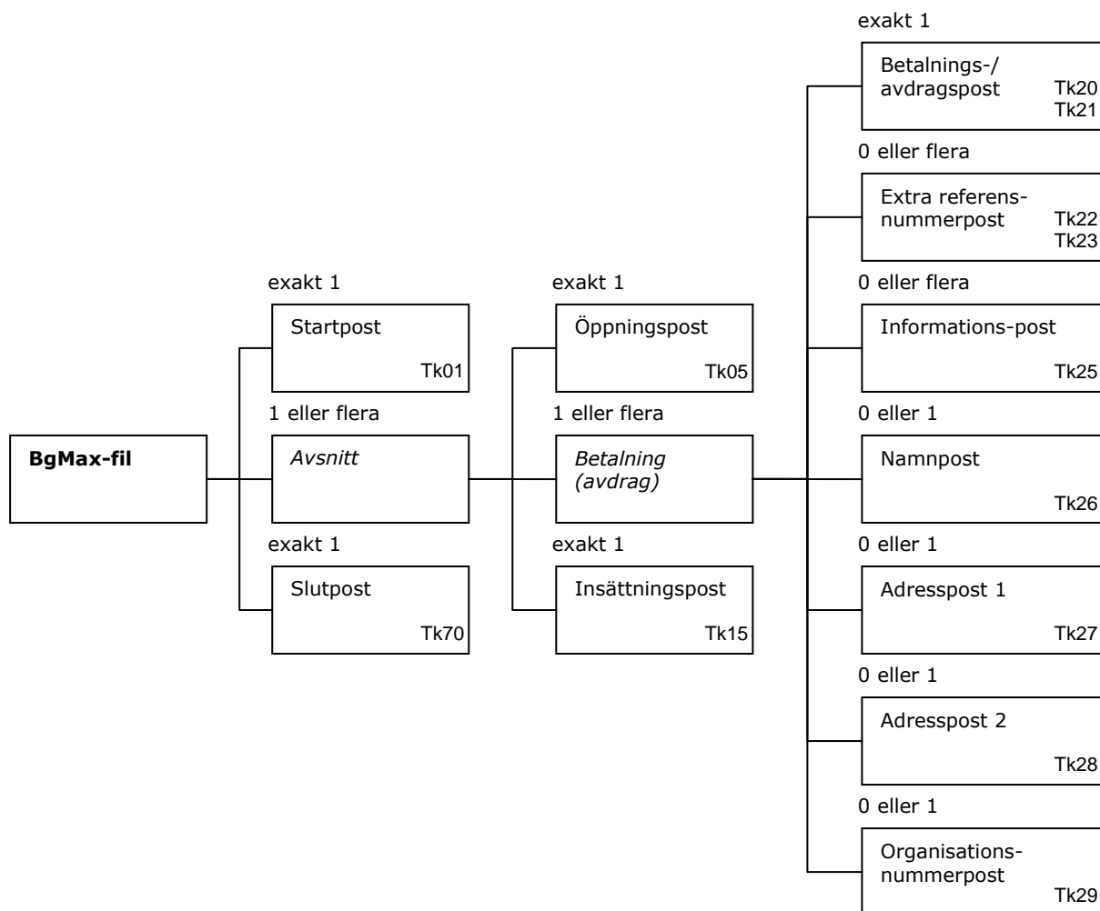
Figur 1: Filstruktur
